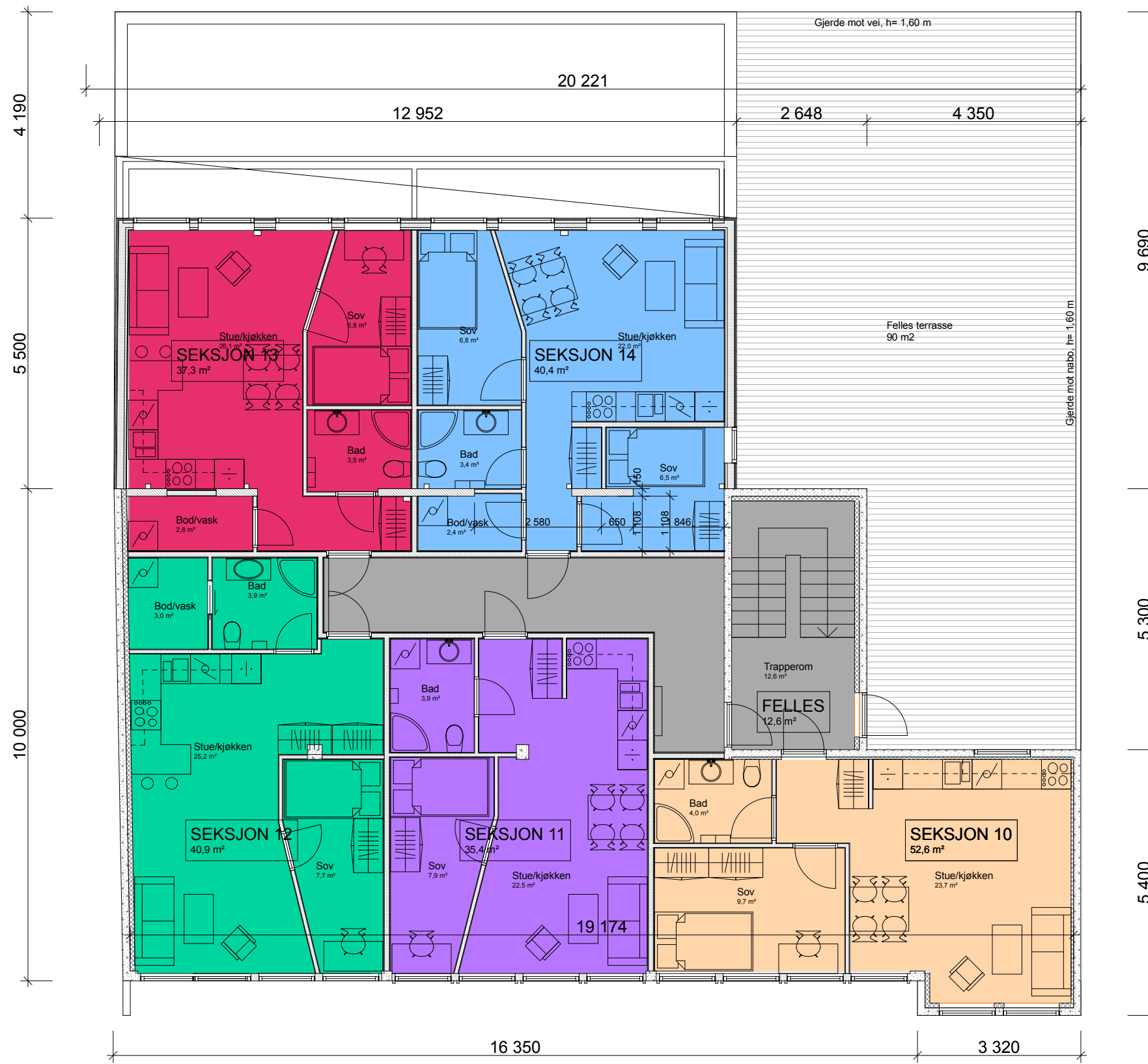
Bruksareal plan 2 227,6 m²
